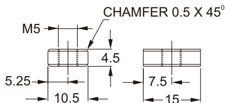
T - NUT
